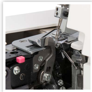
COUPEAU SUPÉRIEUR FACILEMENT ESCAMOTABLE
