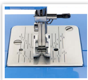
MARQUAGE DÉTAILLÉ DE LA PLAQUE D'AIGUILLE
