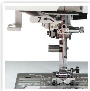
ENFILEUR SUPÉRIEUR DE L'AIGUILLE AVEC 7 GUIDES-FIL
